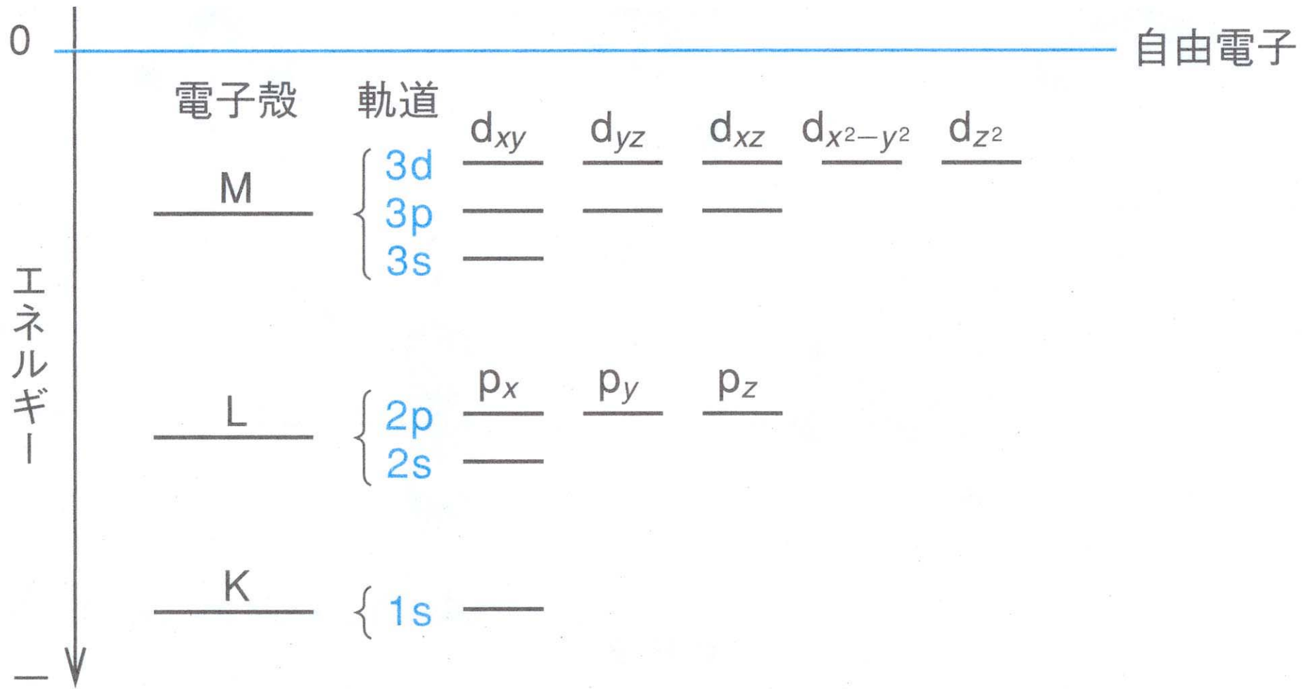
電子殻のエネルギーと軌道のエネルギーの関係
