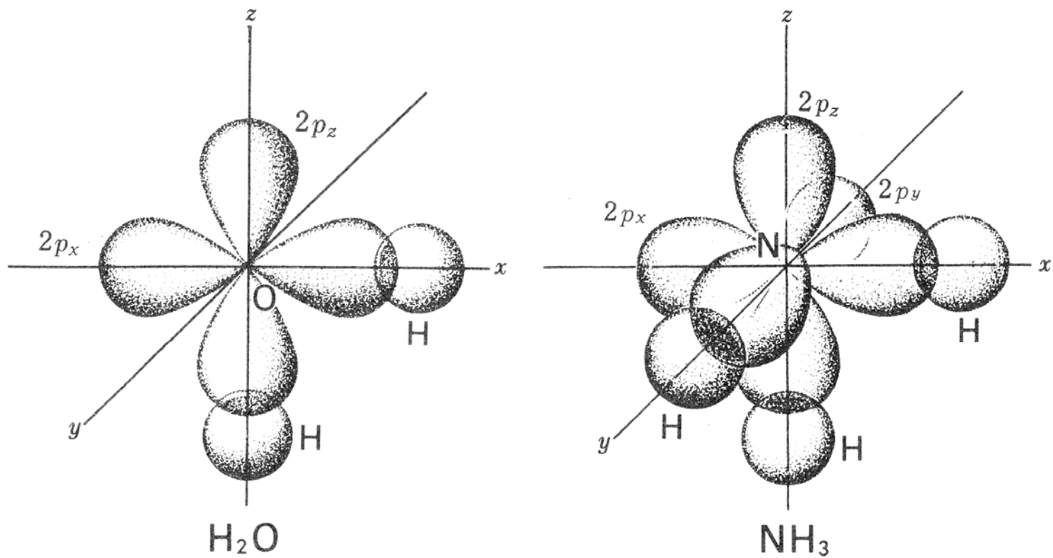
酸素および窒素原子の不对電子のオービタル
