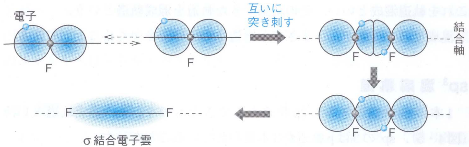
フッ素分子のできる過程
