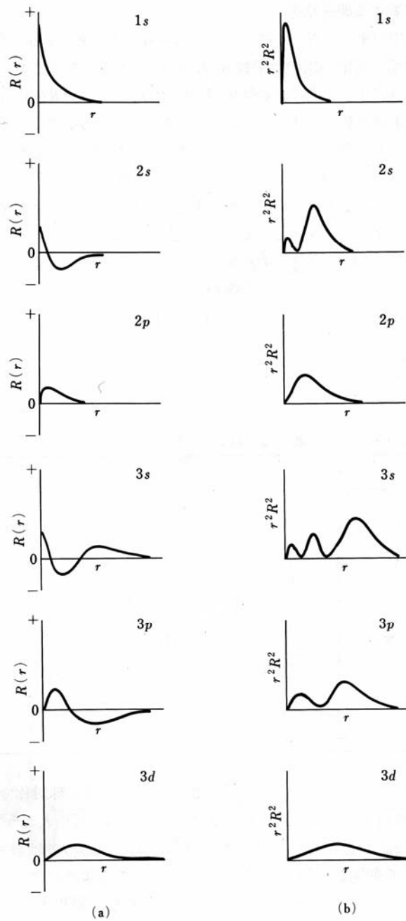
図 2-7 水素類似波動関数のプロット。(a) 原子核からの距離 r に対する動径関数 R(r) 。(b) 原子核からの距離 r に対する確率密度分布関数 r^2R^2 。図によって二つの座標軸の値の範囲が異なることに注意していただきたい。
