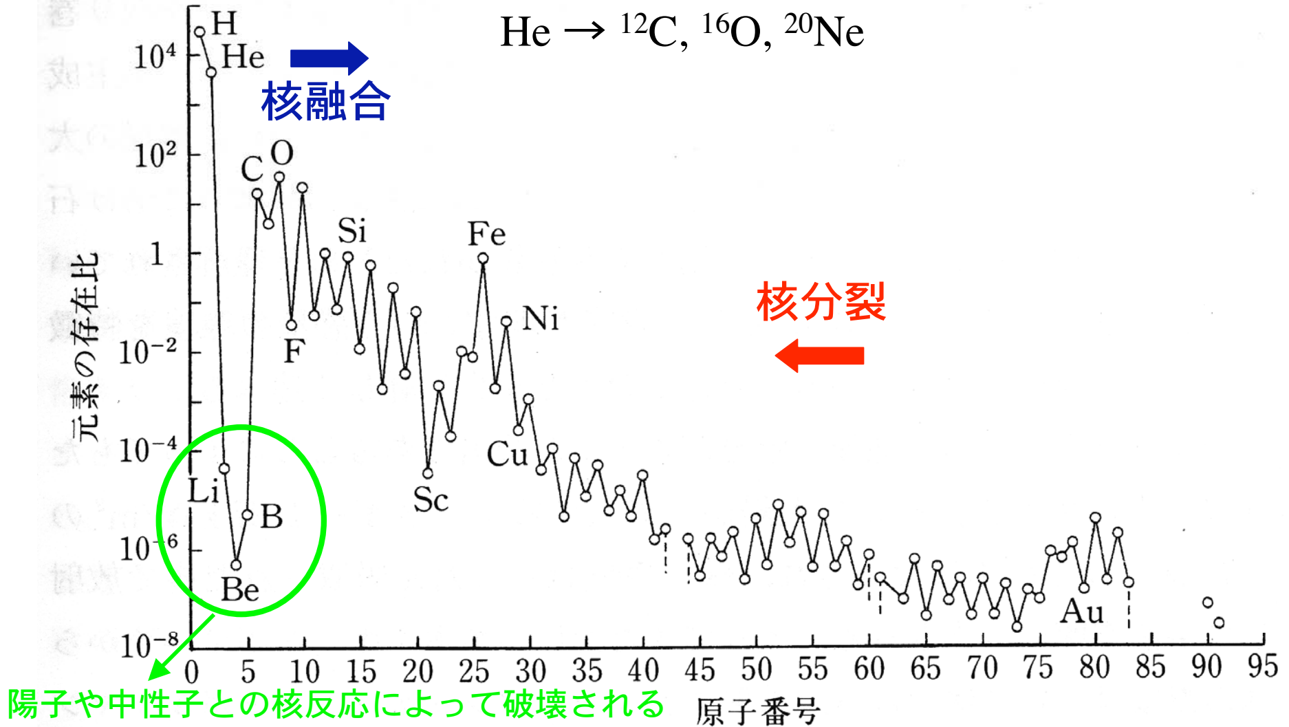
図 1.1 宇宙における元素の存在比. Si を 1 にとってある. [松井義人：地球科学 4 地球の物質科学 III (岩波書店, 1979), p. 265]
