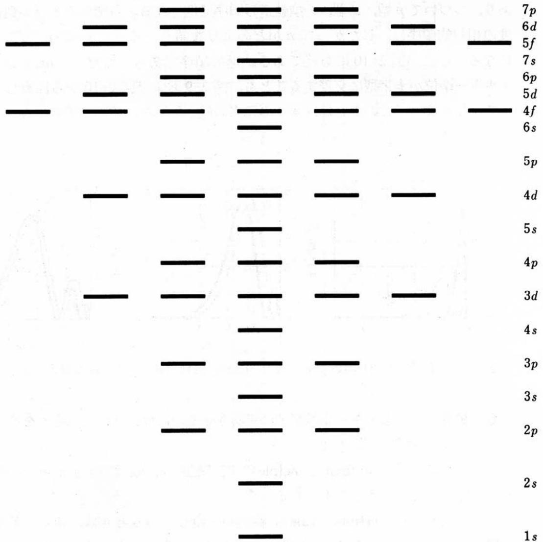
多電子原子における電子収容の順序.
