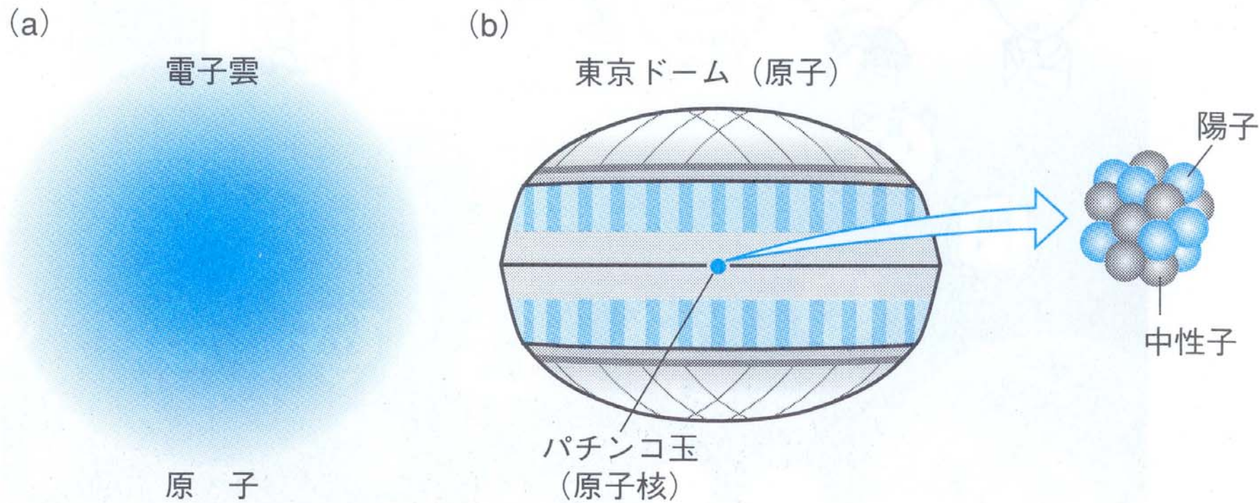
図 1・1 原子の姿. (a) 電子雲, (b) 原子核
