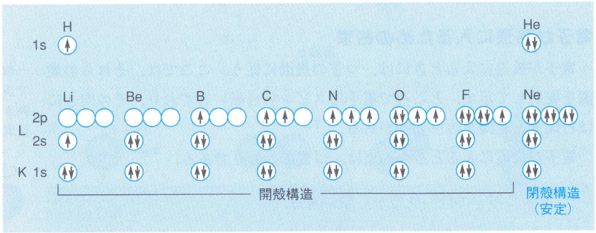
電子配置
