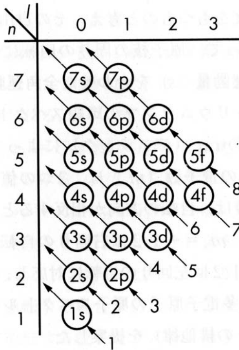
多電子原子における電子収容の順序.
