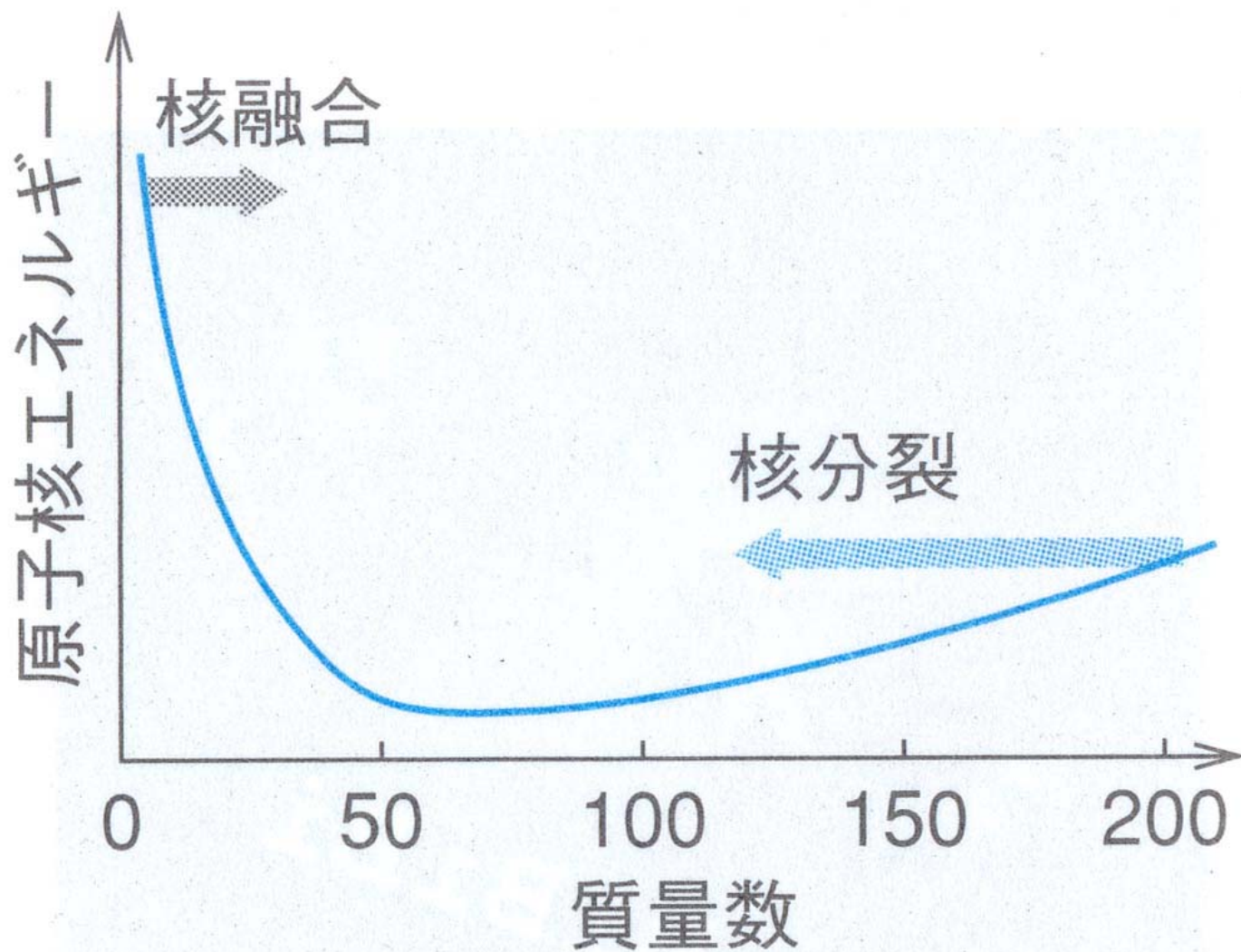
原子核のエネルギーと 質量数の関係
